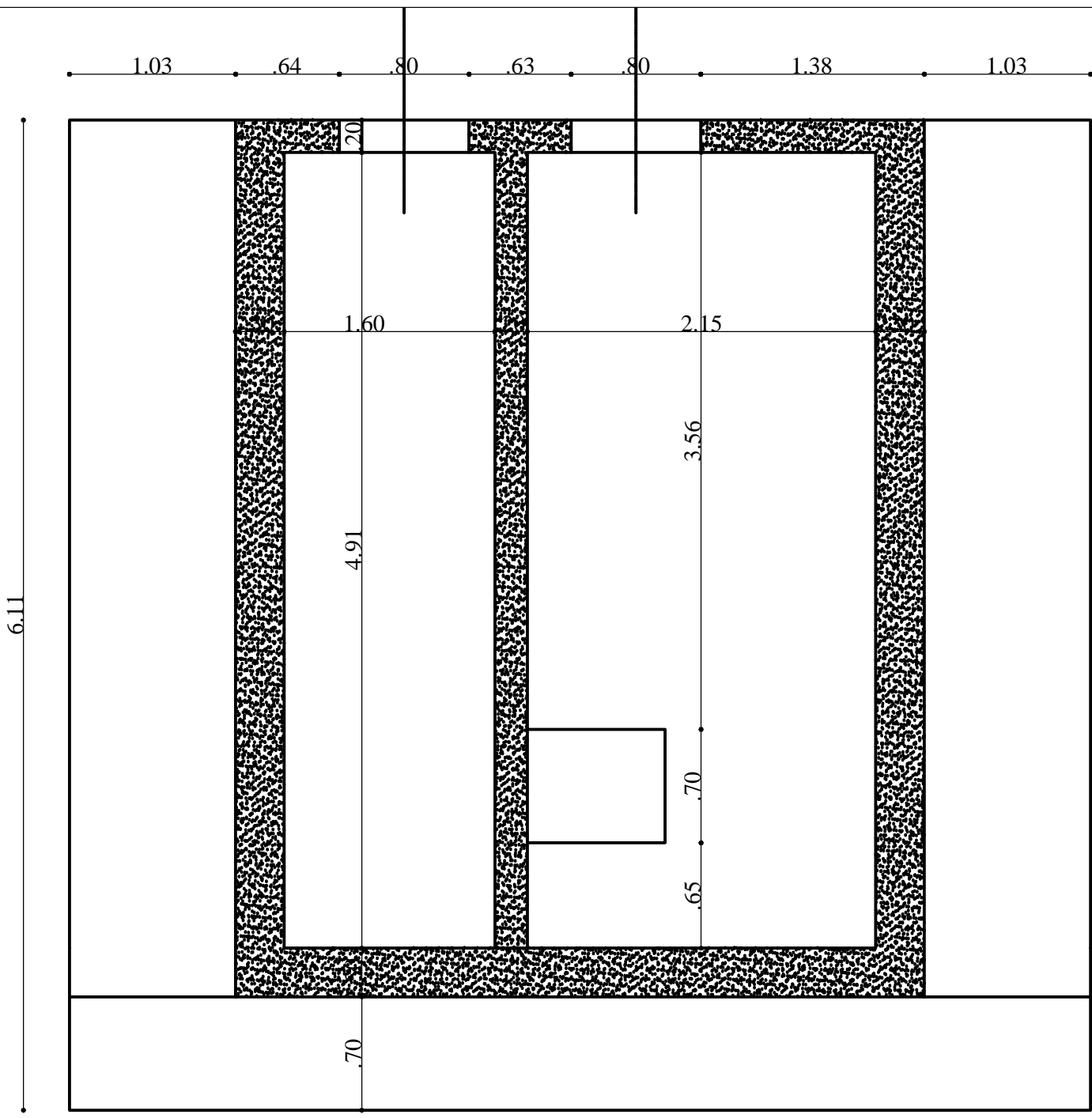
COUPE B-B
